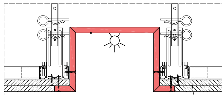
Kształtka FLEXGIPS
