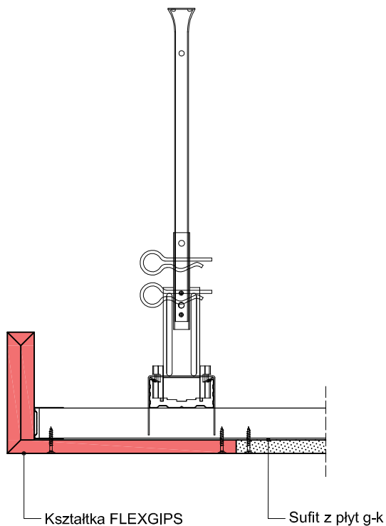
Kształtka FLEXGIPS
